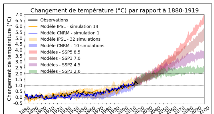
Figure 8. Comme pour la figure précédente, mais avec la prolongation sur le 21 e siècle pour une sélection de quatre scénarios, SSP1 2,6, SSP2 4,5, SSP3 7,0 et SSP5 8,5. Pour chaque scénario, l'enveloppe rassemble l'ensemble des simulations réalisées avec les deux modèles. Période de référence : 1880-1919.
