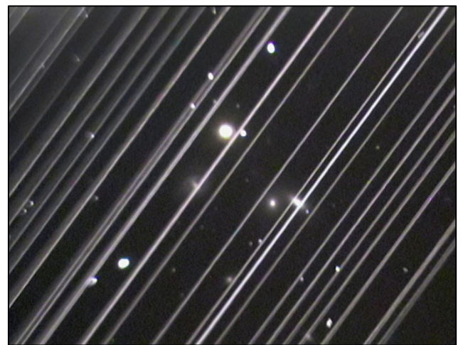
Image du groupe de galaxie NGC 5353/4 réalisé le 25 mai 2019 avec un télescope de l'observatoire Lowell en Arizona (États-Unis). Encore proches les uns des autres moins de deux jours après leur lancement du 23 mai, vingt-cinq des soixante premiers satellites Starlink sont passés dans le champ du détecteur lors de la pose photographique rendant l'image inexploitable. Crédits : Victoria Girgis/Lowell Observatory.
